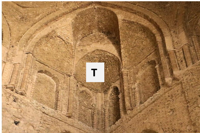
3 Coupole intérieure: trompe de transition
